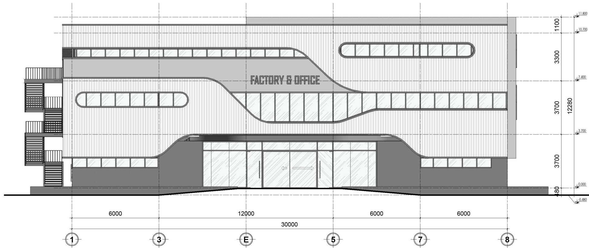
MẶT ĐỨNG TRỤC 1-8
