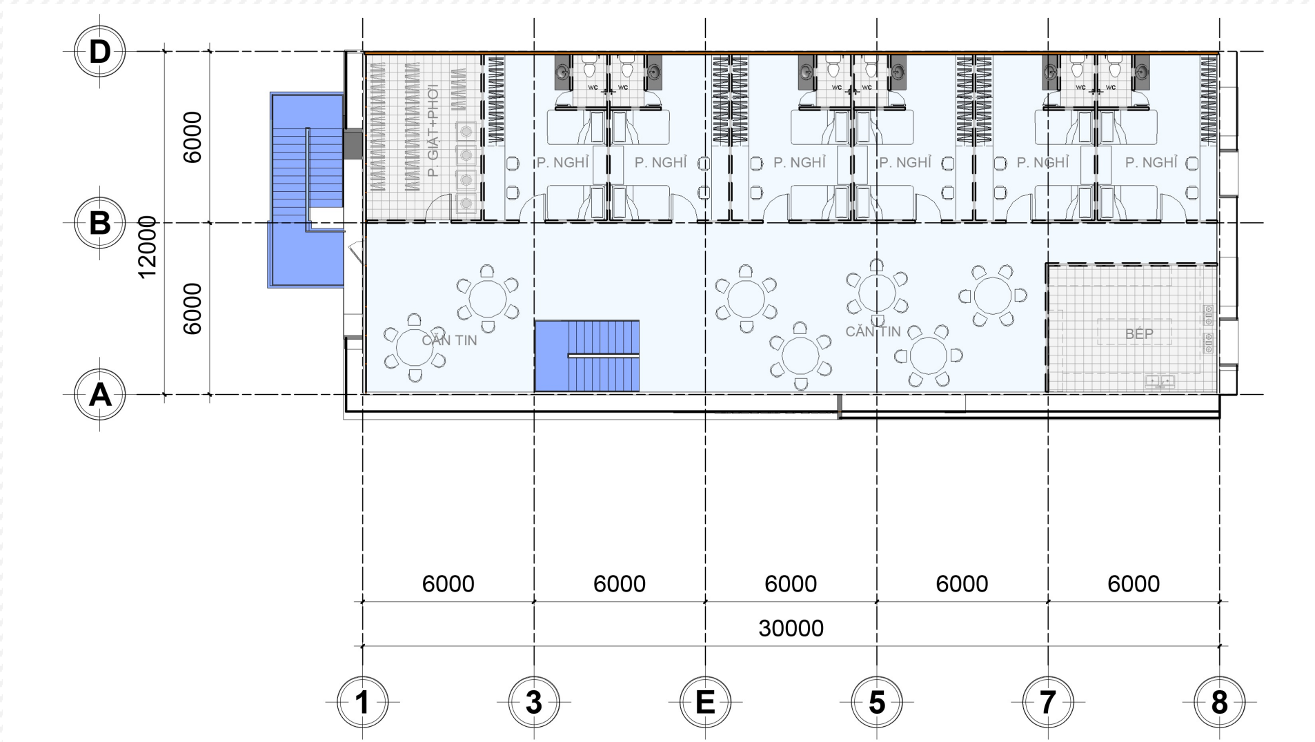
MẶT BẰNG TẦNG 3
