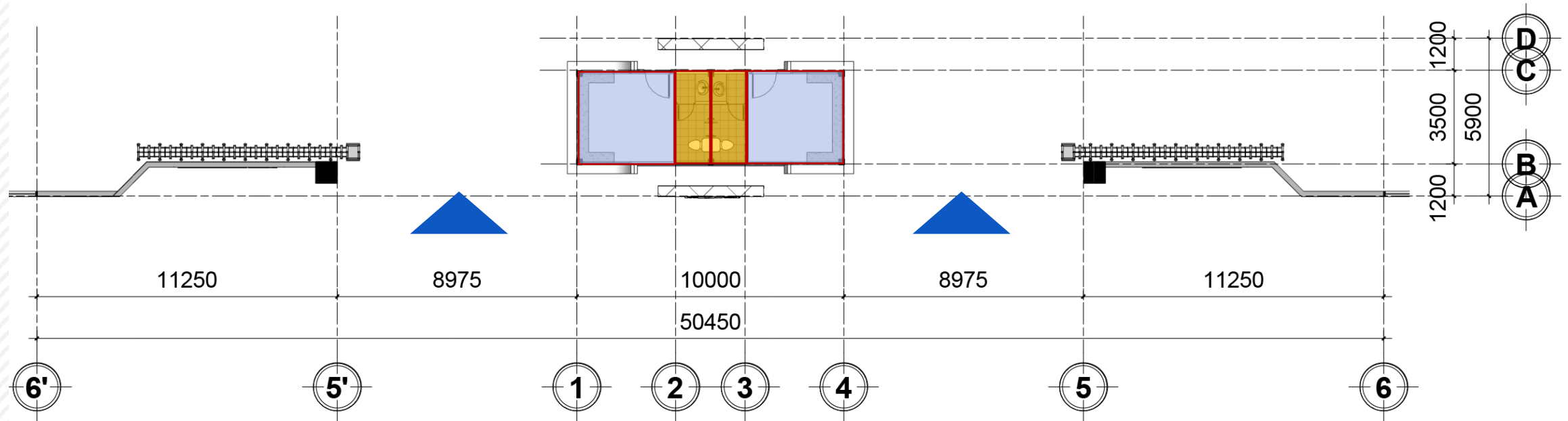
MẶT BẰNG TẦNG 1
