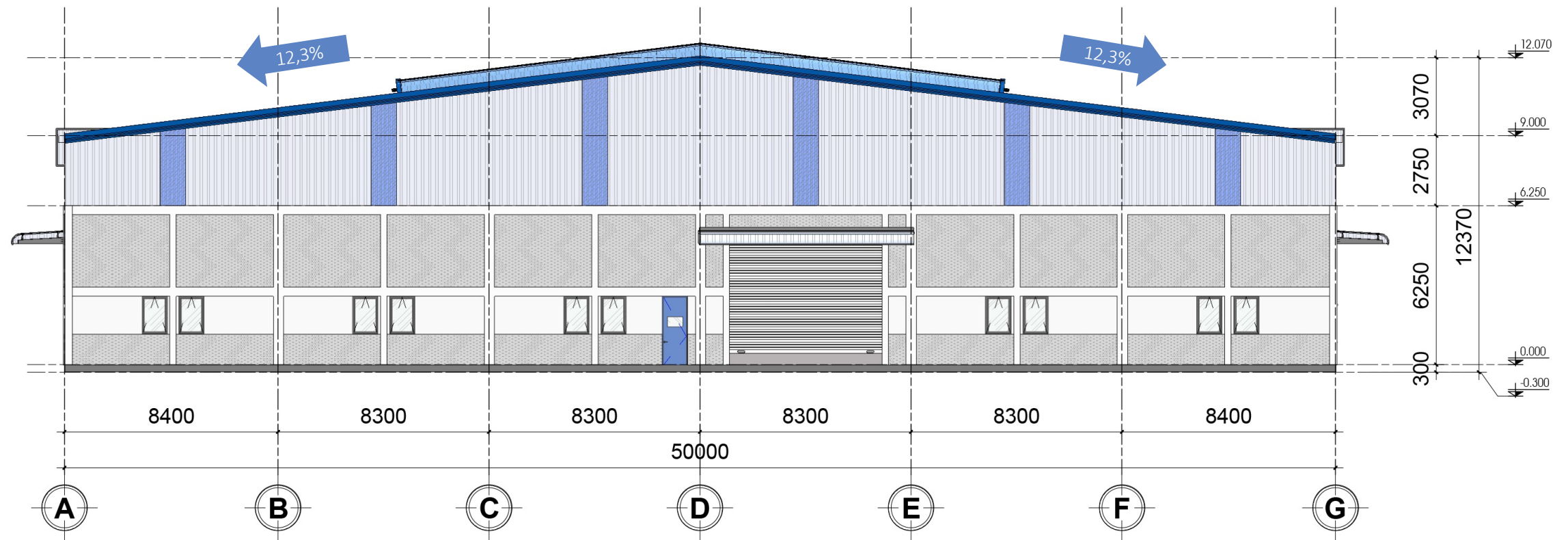
MẶT ĐỨNG TRỤC A-G
