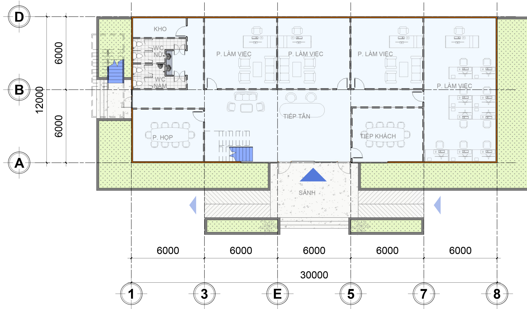
MẶT BẰNG TẦNG 1
