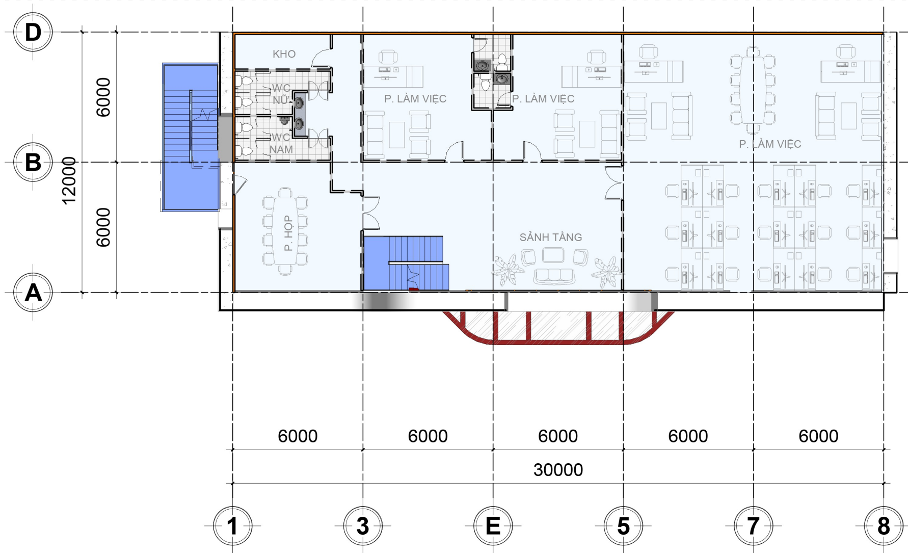
MẶT BẰNG TẦNG 2
