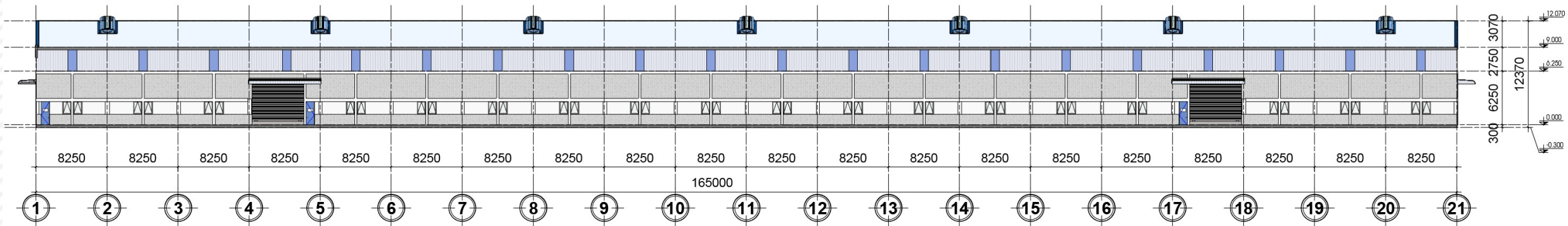
MẶT ĐỨNG TRỰC 1-21
