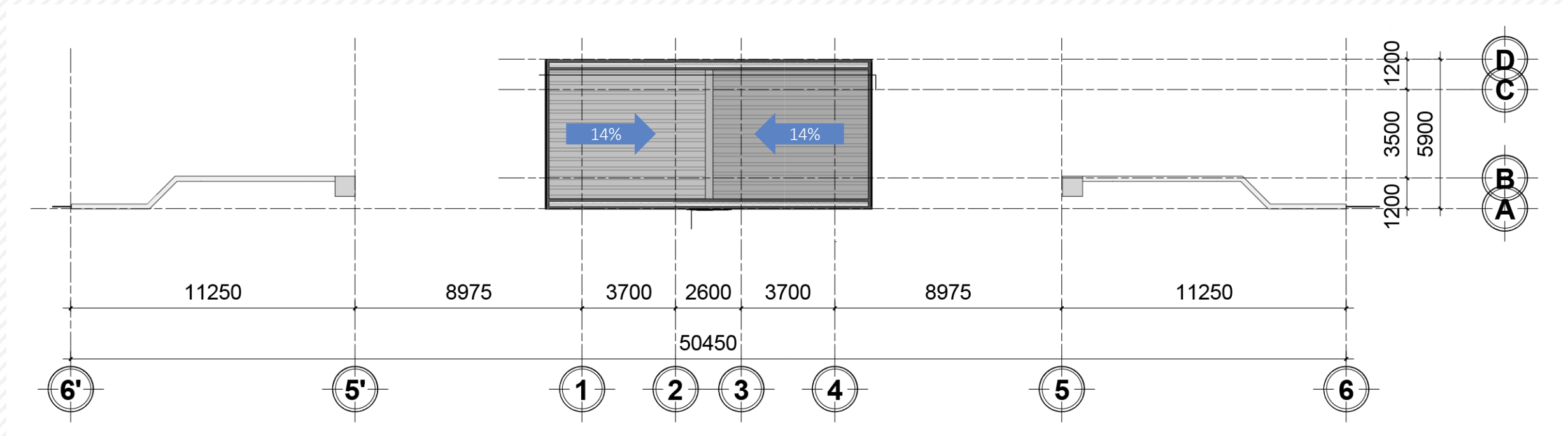
MẶT BẰNG MÁI
