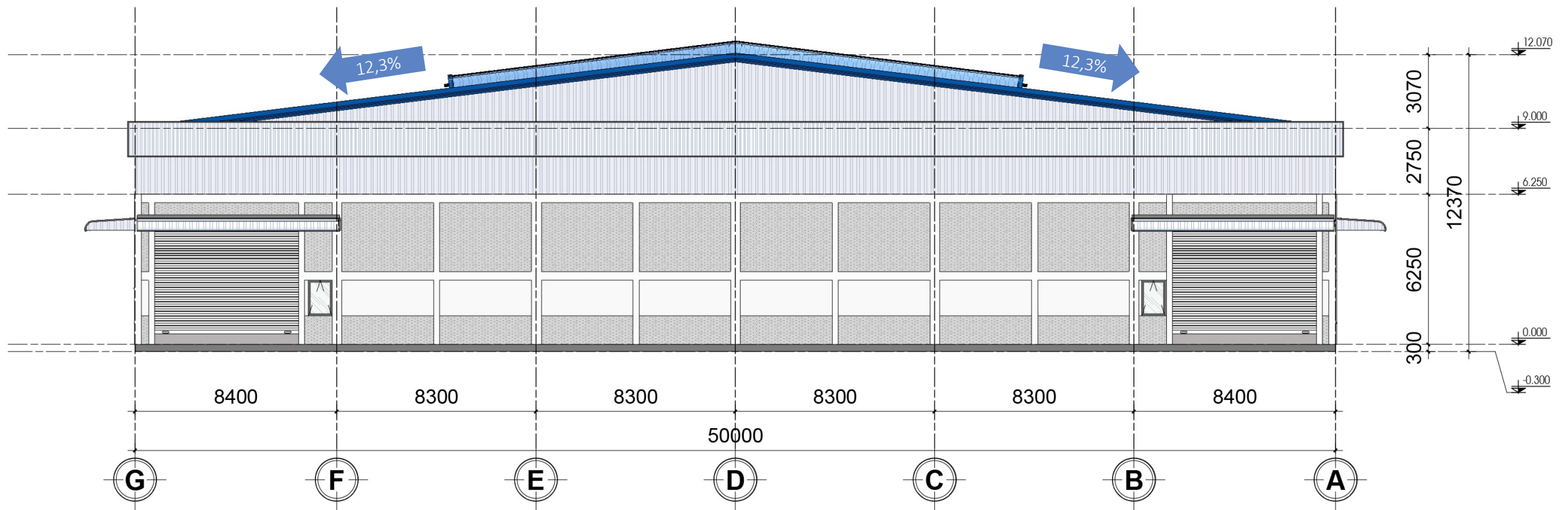
MẶT ĐỨNG TRỤC G-A
