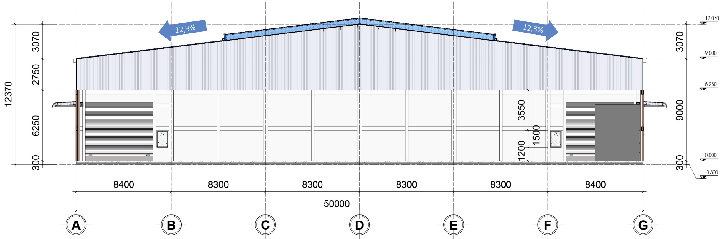
MẶT CẮT XƯỞNG ĐIỂN HÌNH
